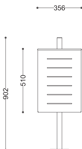
Rzut z frontu
