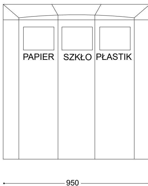
Rzut z frontu
