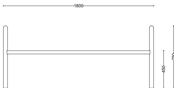
Rzut z frontu
