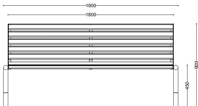
Rzut z frontu
