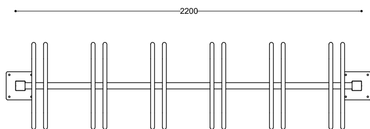
Rzut z góry
