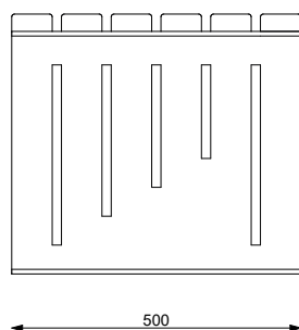
Rzut z boku
