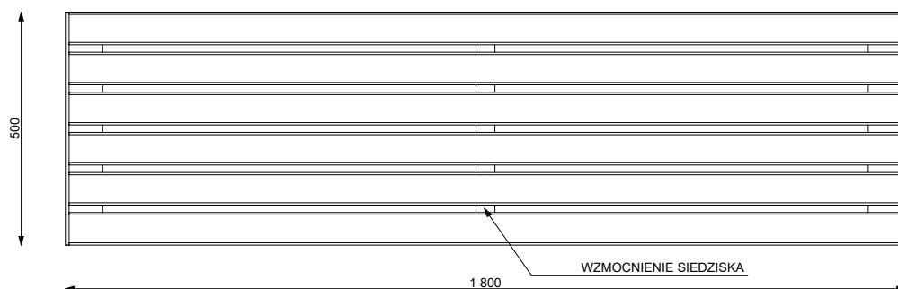
Rzut z góry
