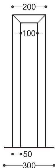
Rzut z frontu
