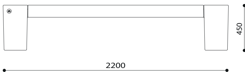
Rzut z frontu
