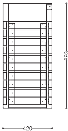
Rzut z frontu
