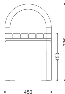
Rzut z boku
